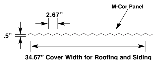
M-Cor
