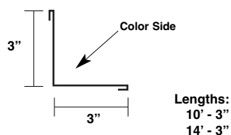
Eave Trim* U-EF
