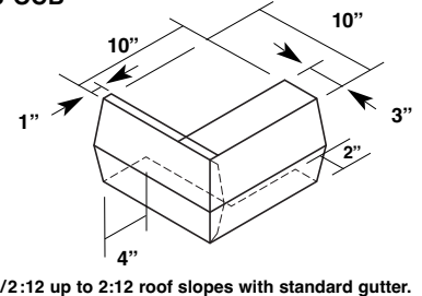
Gutter U-GT
