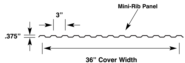
Mini-Rib
