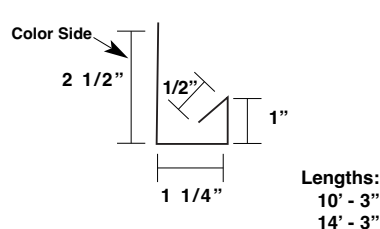
Eave Trim* ITET
