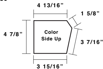
Gutter End Cap UGEC5
