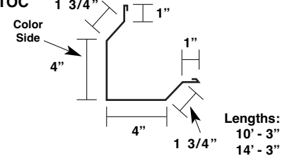
Inside Angle Trim ITIA
