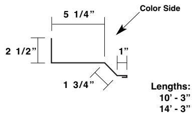
Rake Tie-In Trim ITEW
