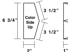
Rake Closure ITREC
