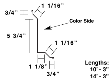
Jamb Trim U-JT
