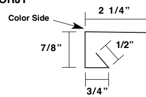
Eave Trim* CORET
