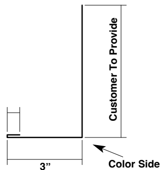
Special Jamb Trim
