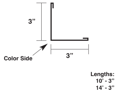
Special Jamb Trim
