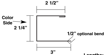
Cap Trim Item #: 38381
