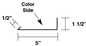
Flared Edge Trim Item #: 38383
